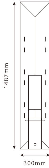
背面
