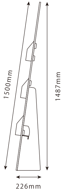
側面
