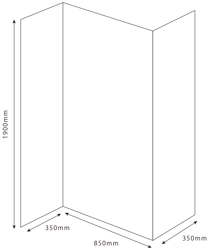
全体図
