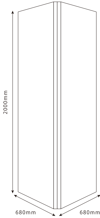
全体図
