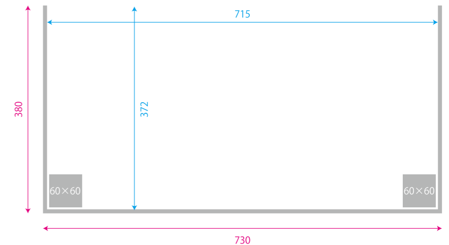
背面スペース寸法図
