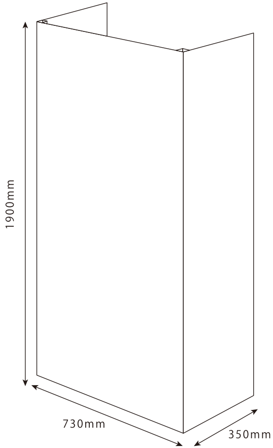
全体図
