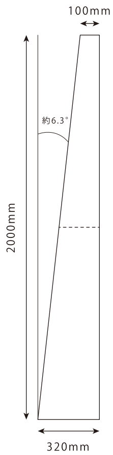
側面
