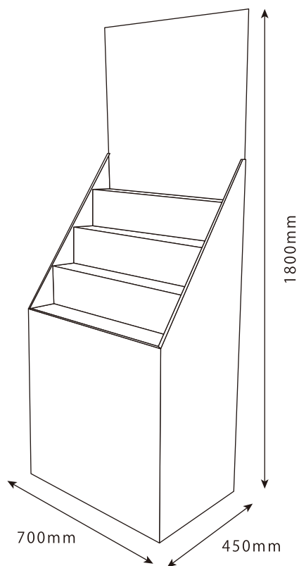
全体図
