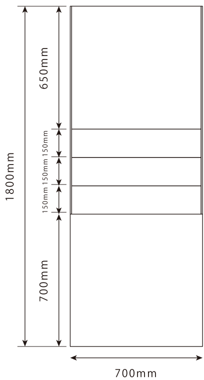
正面
