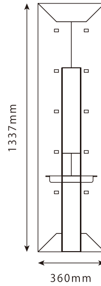
背面
