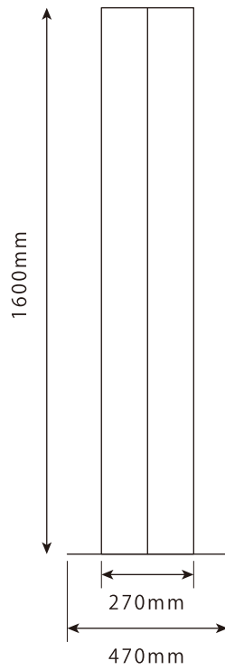
背面
