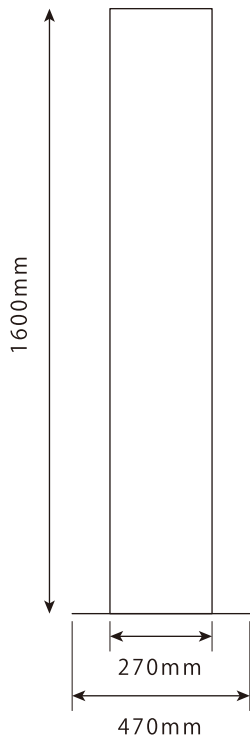
正面・側面
