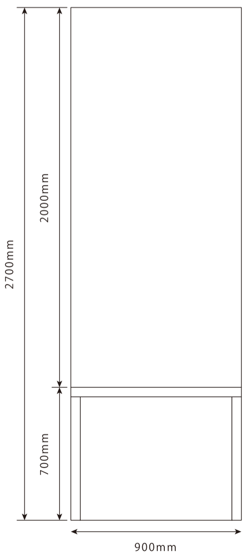
正面
