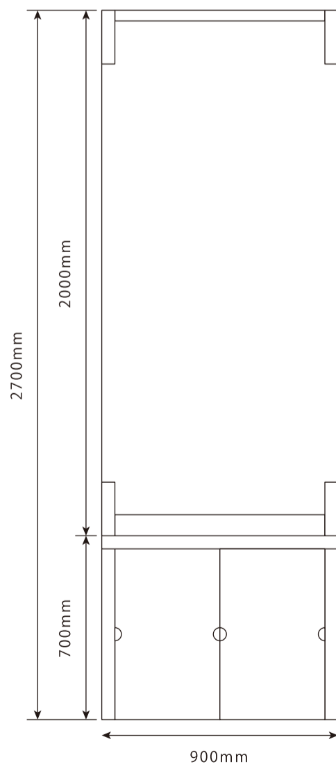
背面
