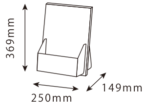
全体図
