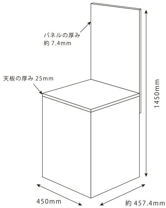
全体図（正面側）
