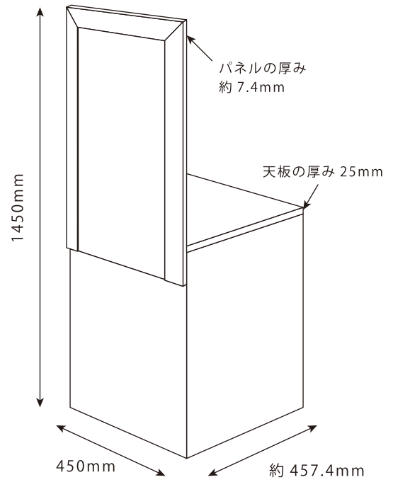
全体図（背面側）
