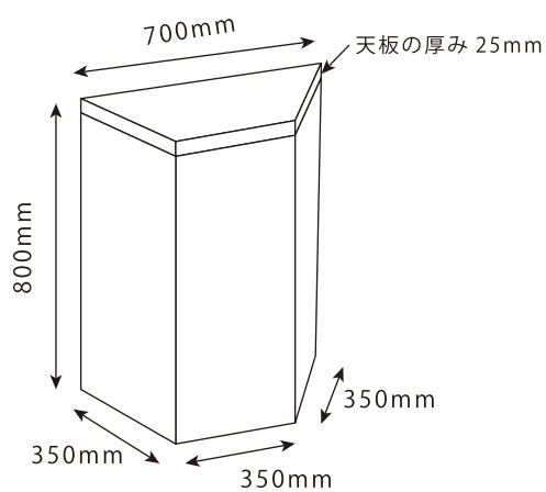
全体図
