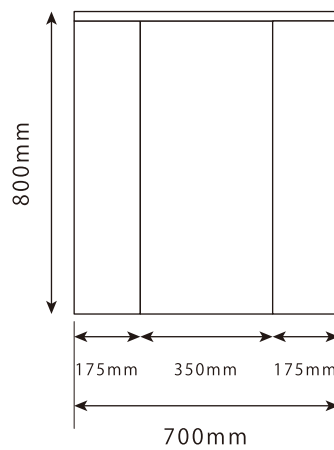
背面
