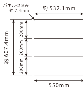
上面
