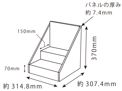
全体図（正面側）
