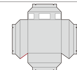
本体板 / 大 (×1)
