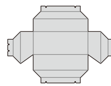
本体板 / 小 (×1)
