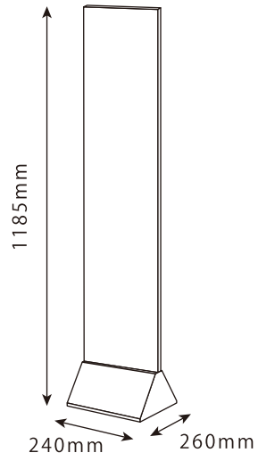
全体図
