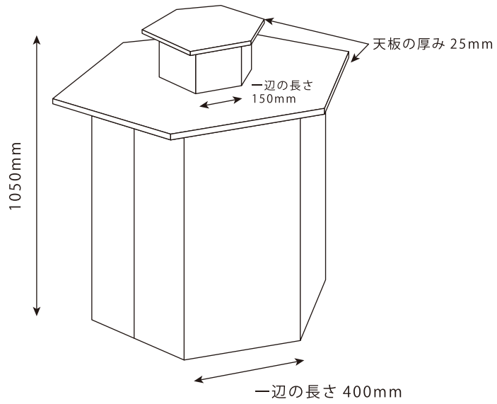
全体図
