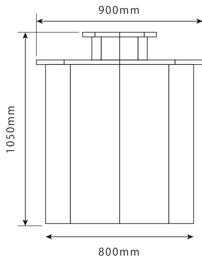
側面
