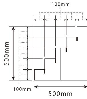
側面
