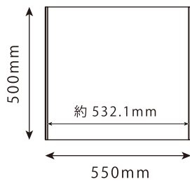
背面
