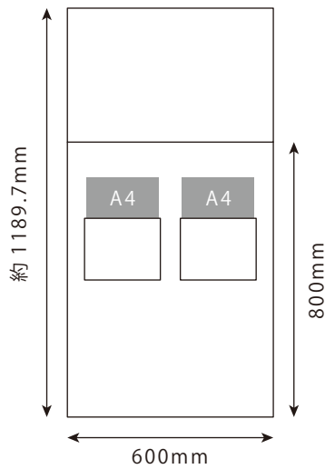
正面
