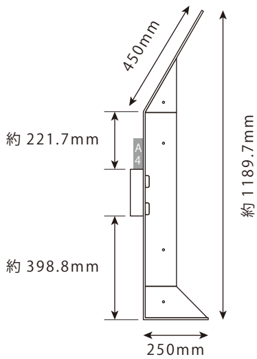
側面
