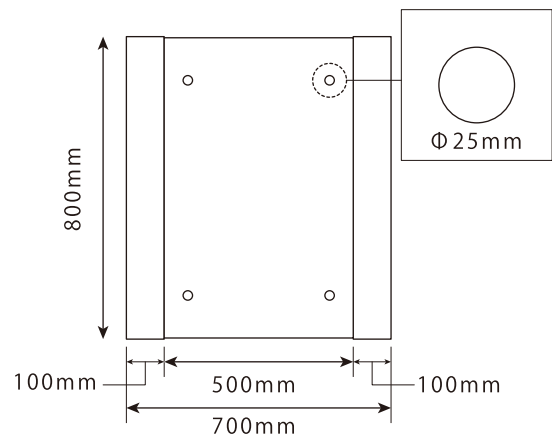
背面
