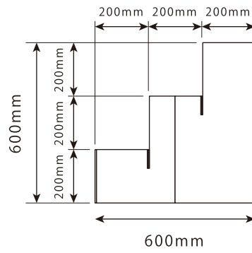
側面
