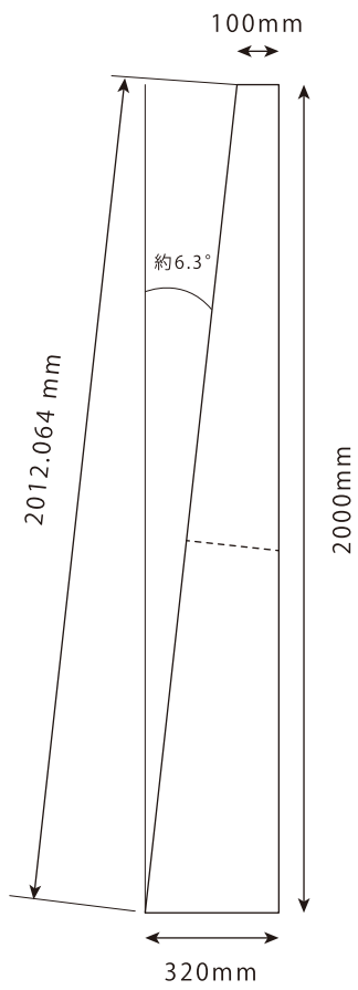
側面
