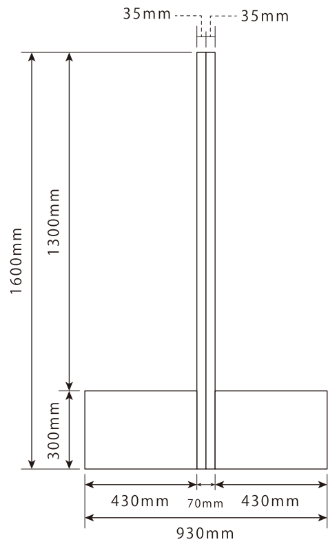
側面
