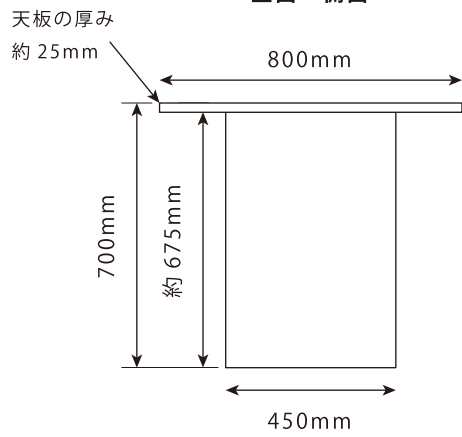
正面・側面
