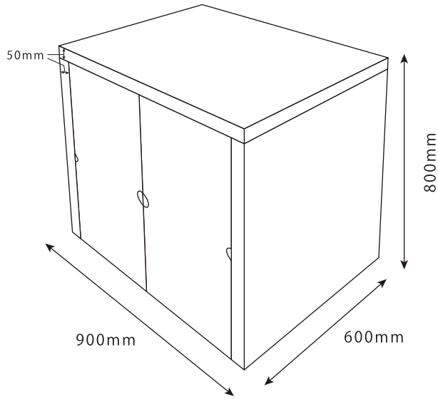
全体図
