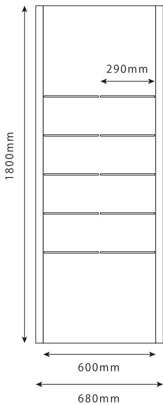
正面・側面
