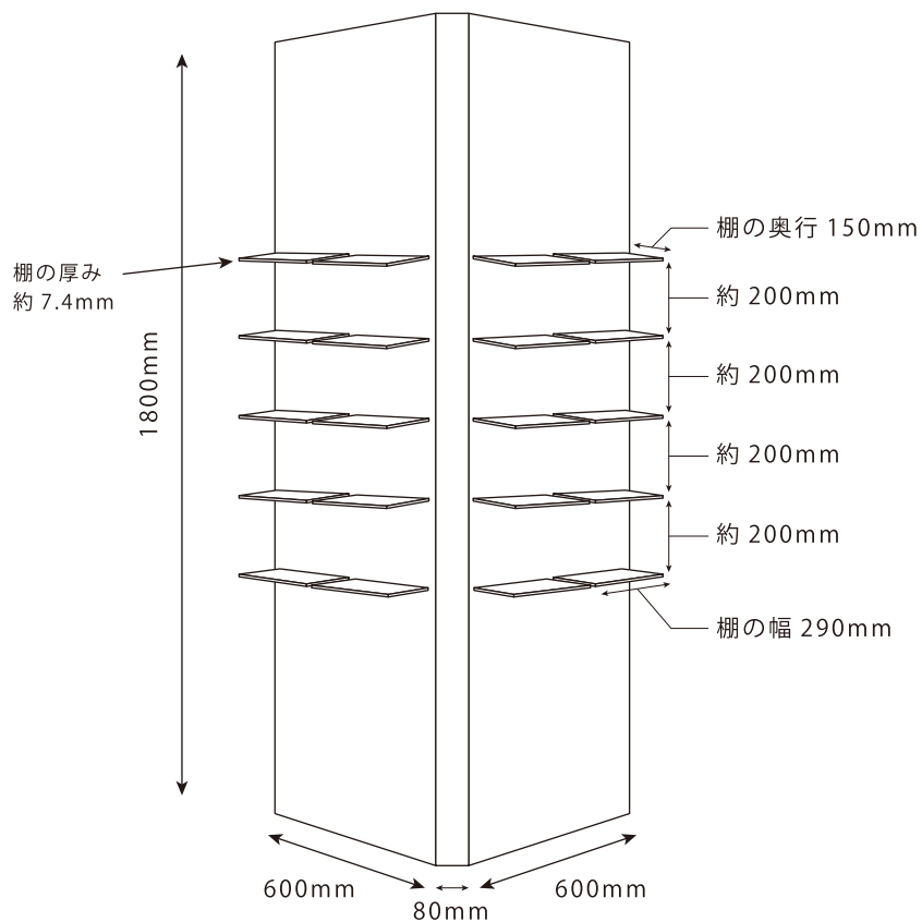
全体図
