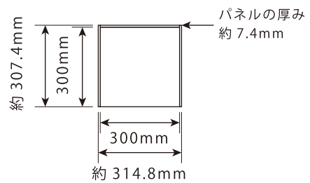
上面
