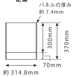
正面
