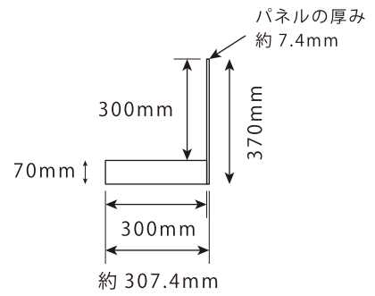
側面 (内寸)
