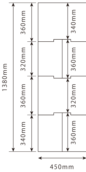
正面
