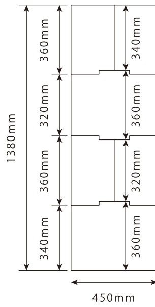
背面
