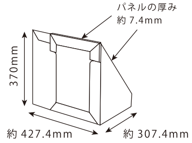
全体図 (背面側)
