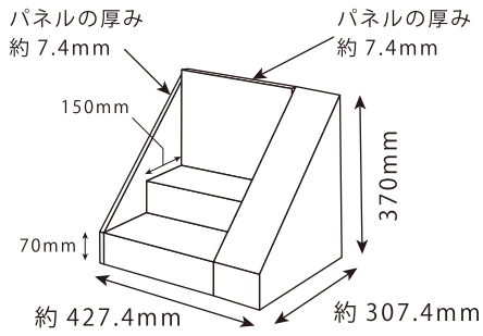
全体図 (正面側)
