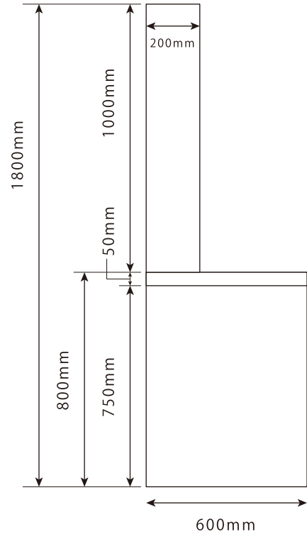
側面
