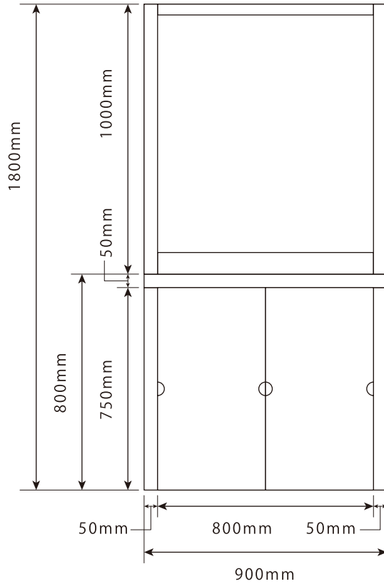
背面
