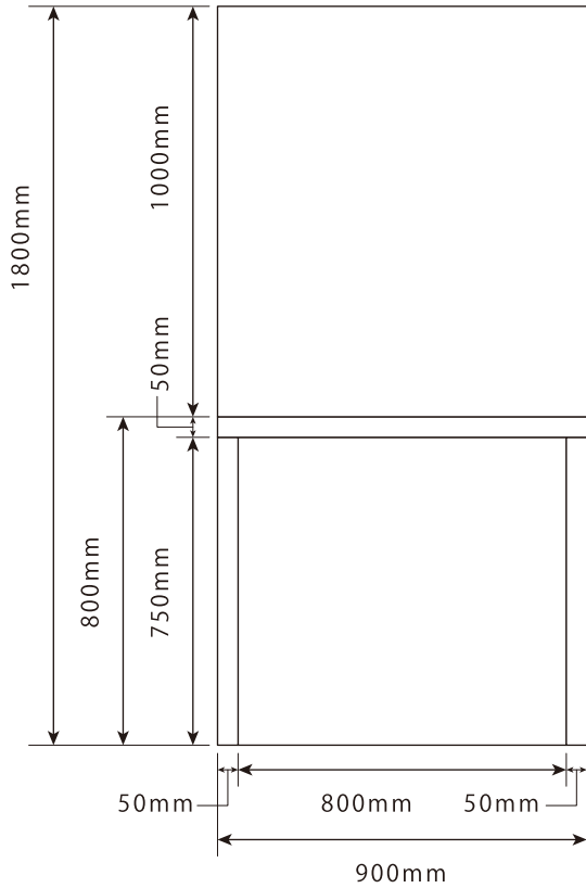
正面
