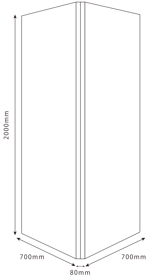
全体図
