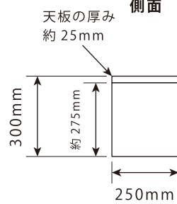
側面
