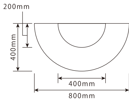
天面 (2 段)
