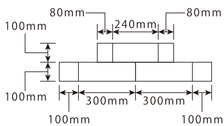
背面 (2 段)
