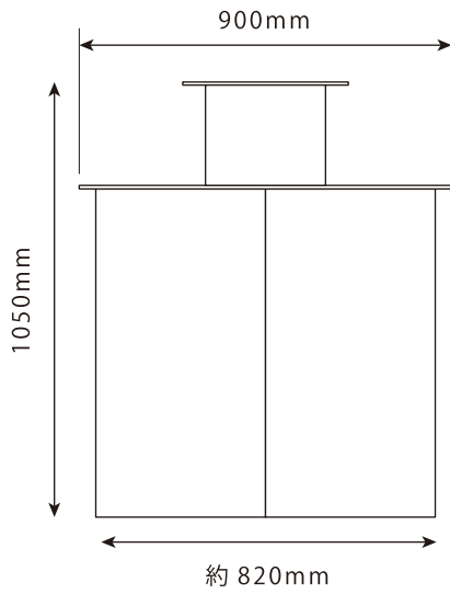
側面
