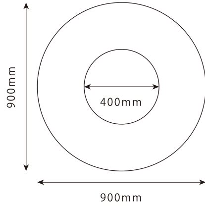
上面
