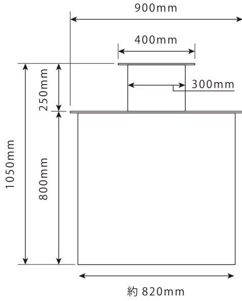
正面
