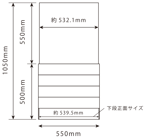
正面
