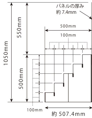
側面
