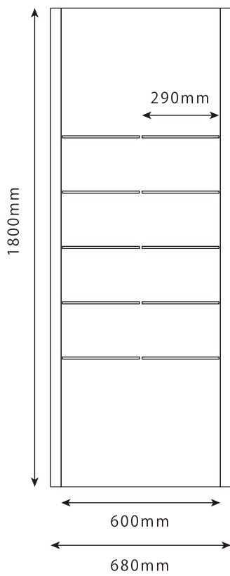
正面・側面
