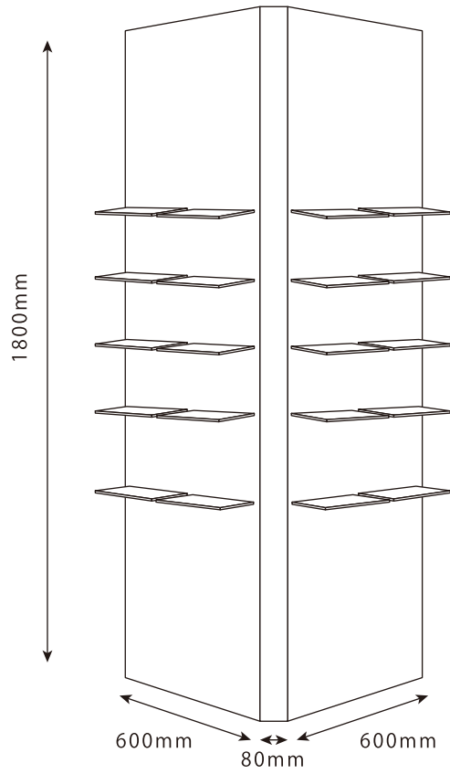
全体図
