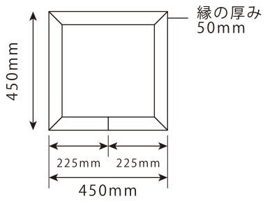
正面・背面
