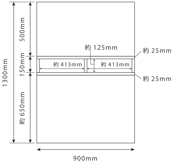
正面
