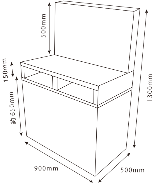
全体図
