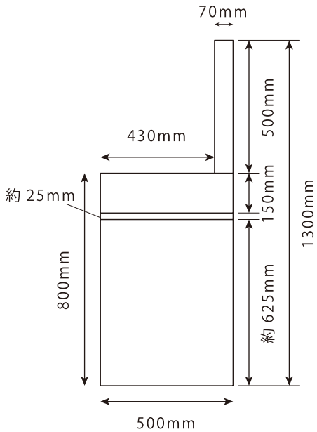
側面
