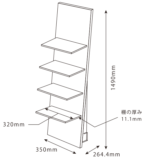
全体図
