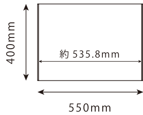
背面
