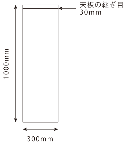
正面・側面
