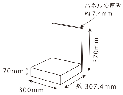
全体図 (正面側)
