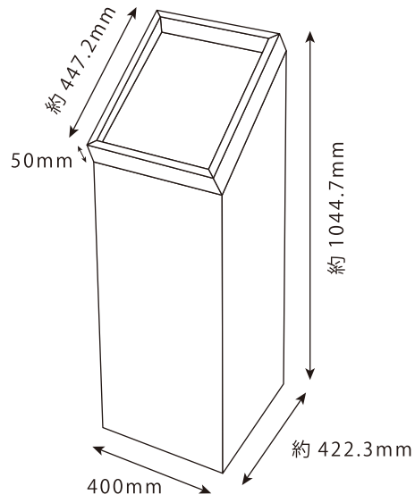
全体図
