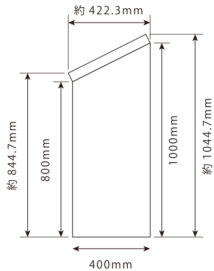
側面
